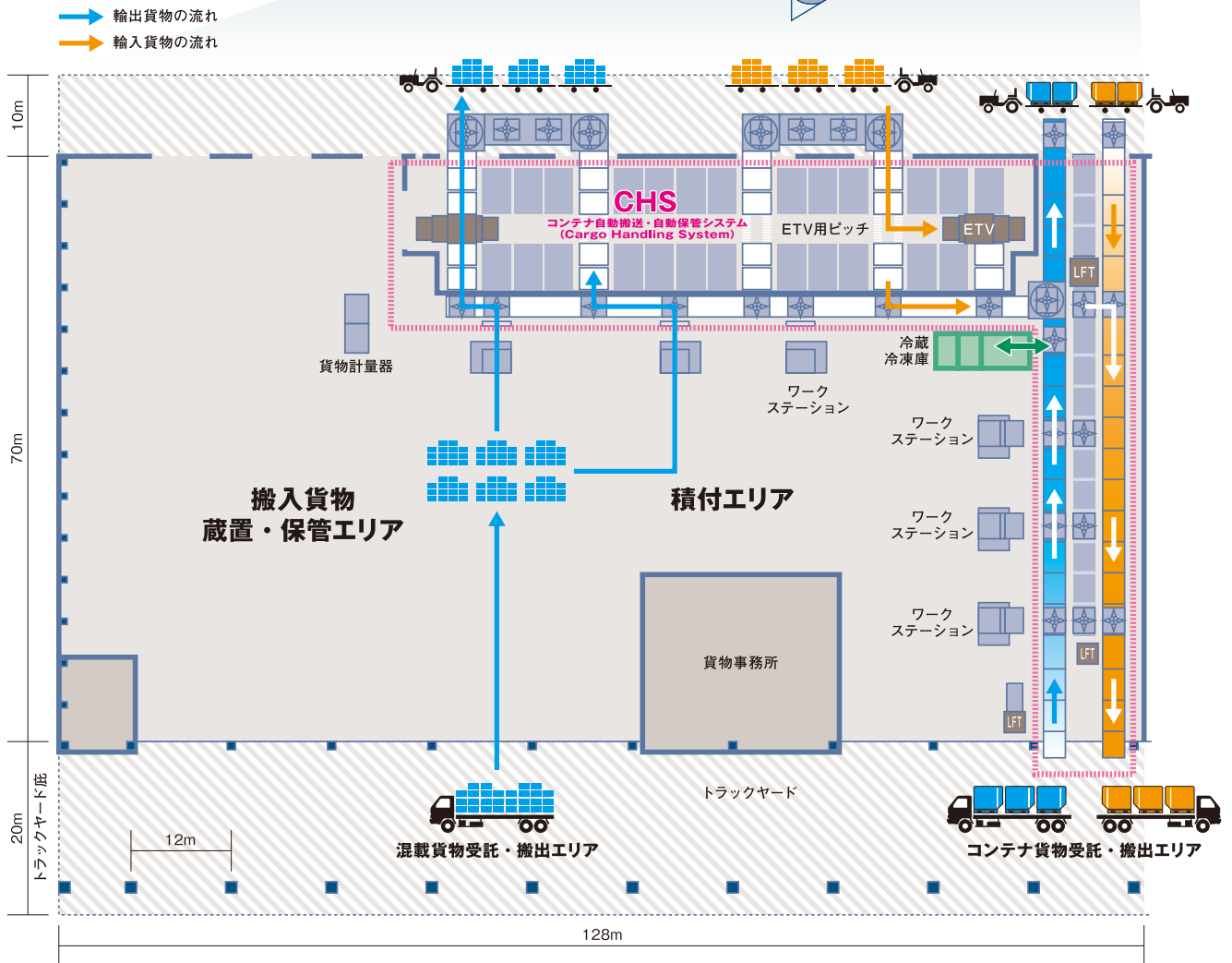
コンテナ自動搬送・自動保管システム
